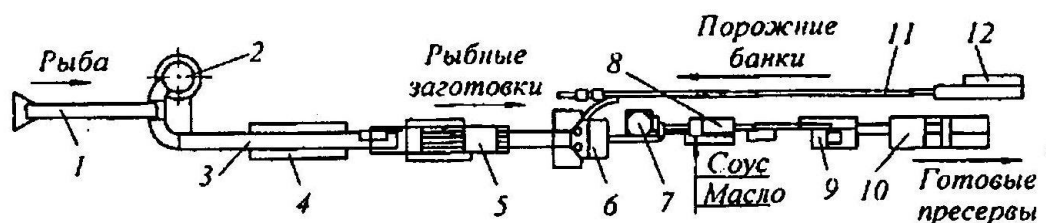
Рисунок 13 - Машинно-аппаратурная схема линии производства рыбных пресервов
