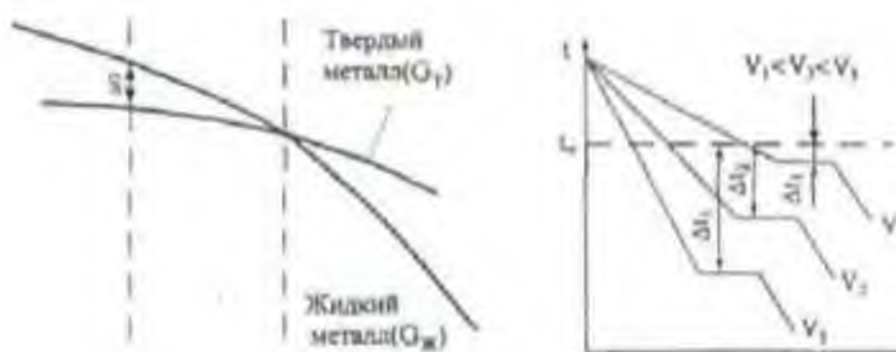
Рис.5.1 Изменение энергии Гиббса металла в жидком ( G_{ж} ) и твердом ( G_{т} ) состояниях в зависимости от температуры
