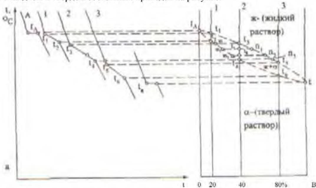
Диаграмма состояния для случая неограниченной растворимости компонентов A и B в жидком и твердом состояниях: а - кривые охлаждения; б - диаграмма состояния
