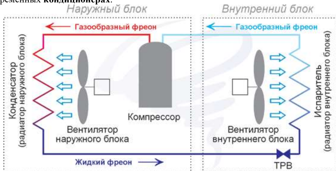
Рисунок 1. Схема сплит-системы
