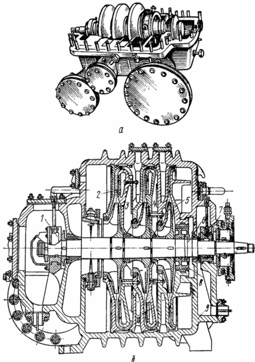
Рис. 31. Фреоновый турбокомпрессор: а — общий вид со снятой крышкой и заглушками на штуцерах, б — продольный разрез; 1 — опорно-упорный подшипник. 2 — диффузор. 3, 4, 5 — рабочие колеса, 6 — вал, 7 — опорный подшипник, 8 — думмис, 9 — корпус, 10 — обратный направляющий аппарат
