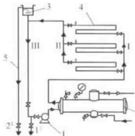
Рис. 2. Схема охлаждения хладоносителем с закрытыми охлаждающими приборами и закрытым испарителем: 1-насос; 2-испаритель; 3-расширительный бак; 4-охлаждение батареи; 5-переливная труба; 1 1 , 2 1 - задвижки.
