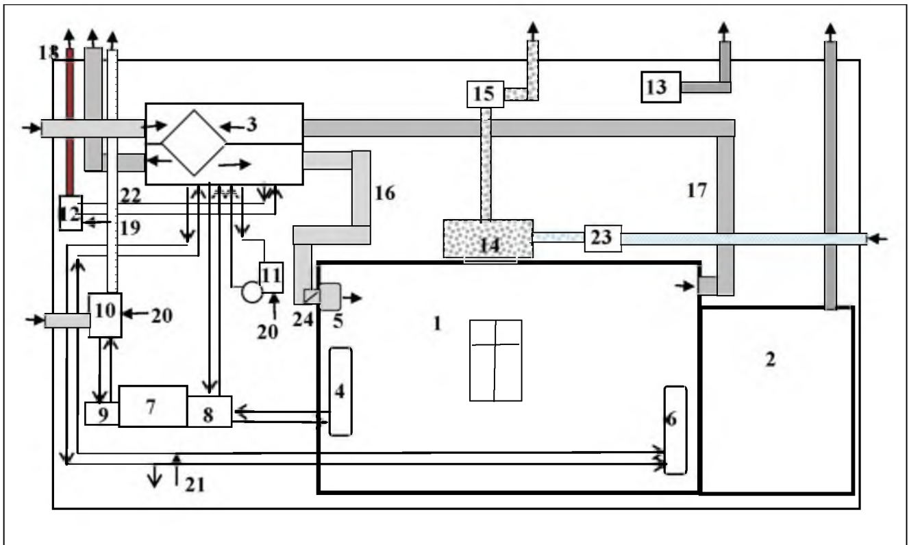
Рисунок 1 Принципиальная схема системы отопления, вентиляции и кондиционирования воздуха в жилом доме
